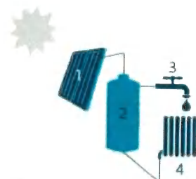
1 Zonnecollector | 2 Opslagvat zonneboiler | 3 Sanitair warm water | 4 Afgifte element voor ruimtewarming (radiator)
